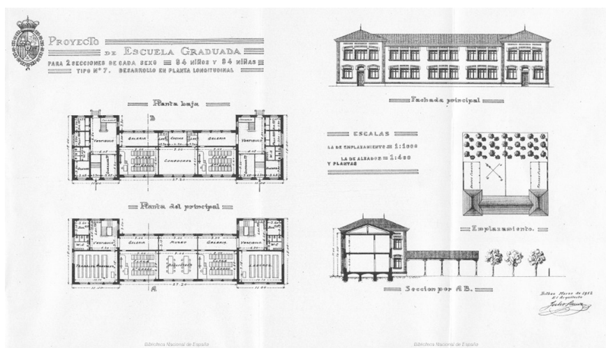
Fig. 6. Proyecto de Escuelas graduadas para dos secciones de cada sexo. Tipo 7. Planos Modelos de Escuelas Graduadas con Presupuestos Reducidos . Edición oficial. Madrid, Imprenta Nacional del Colegio de Sordomudos y Ciegos, 1912.
