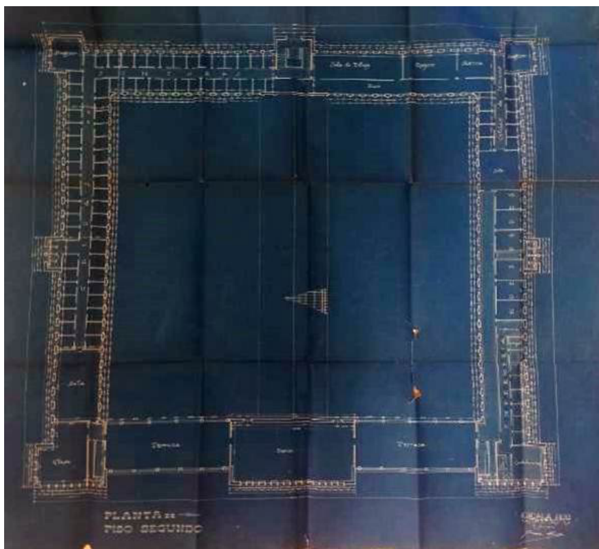
Fig. 16. Planta segundo piso. Seminario de Albelda. Archivo Calasancio. Padres Escolapios Madrid.
