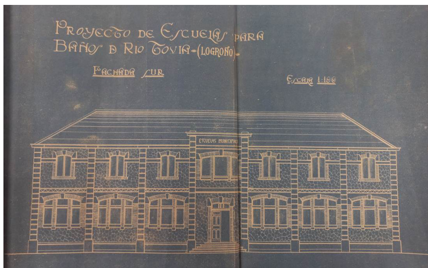
Fig. 2. Plano de la fachada principal al sur. Escuelas de Baños de Río Tobía. Fotografía, ICV.
