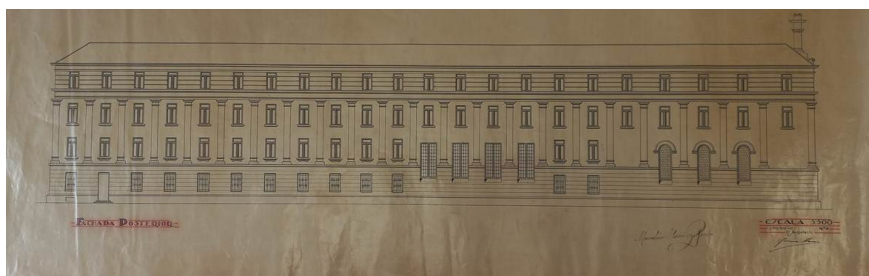
Fig. 13. Fachada posterior. Colegio Padres Escolapios. Fermín Álamo, 1928. AML.
