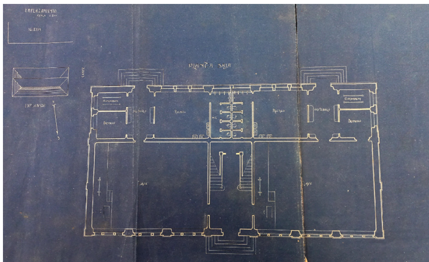
Fig. 4. Planta baja. Escuelas de Baños de Río Tobía. Fotografía, ICV.
