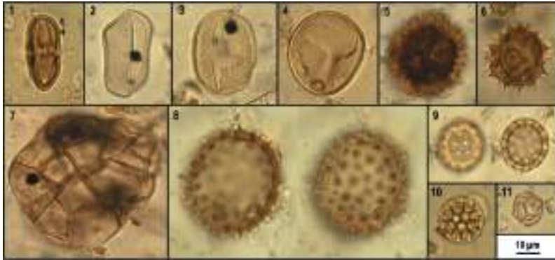
Figura 1. Principales granos de polen. 1. Apiaceae; 2, 3. Liliaceae/Amaryllidaceae; 4. Malvaceae; 5. Poaceae; 6. Fabaceae-Mimosoideae; 7. Asteraceae-Cichorioideae; 8. Asteraceae subf. Asteroideae; 9. Amaranthaceae; 10. Gomphrena ; 11. Alternanthera .
